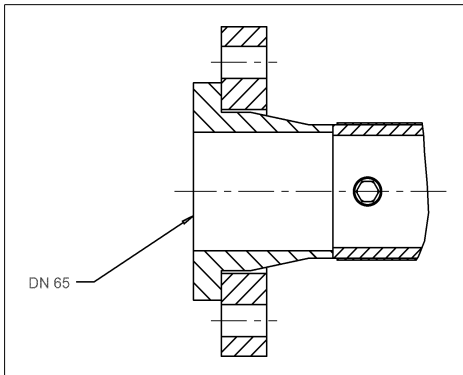
Abb. 7: Anschluss des Einzelenthärters
