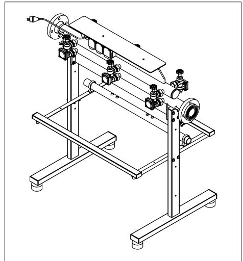
Abb. 9: Verteiler und Gestell i-soft 10, 15, 20 TGA (Beispiel i-soft 15 TGA)
