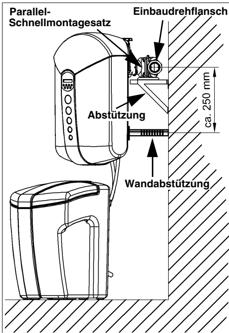
Abb. 5: Abstützungselemente
