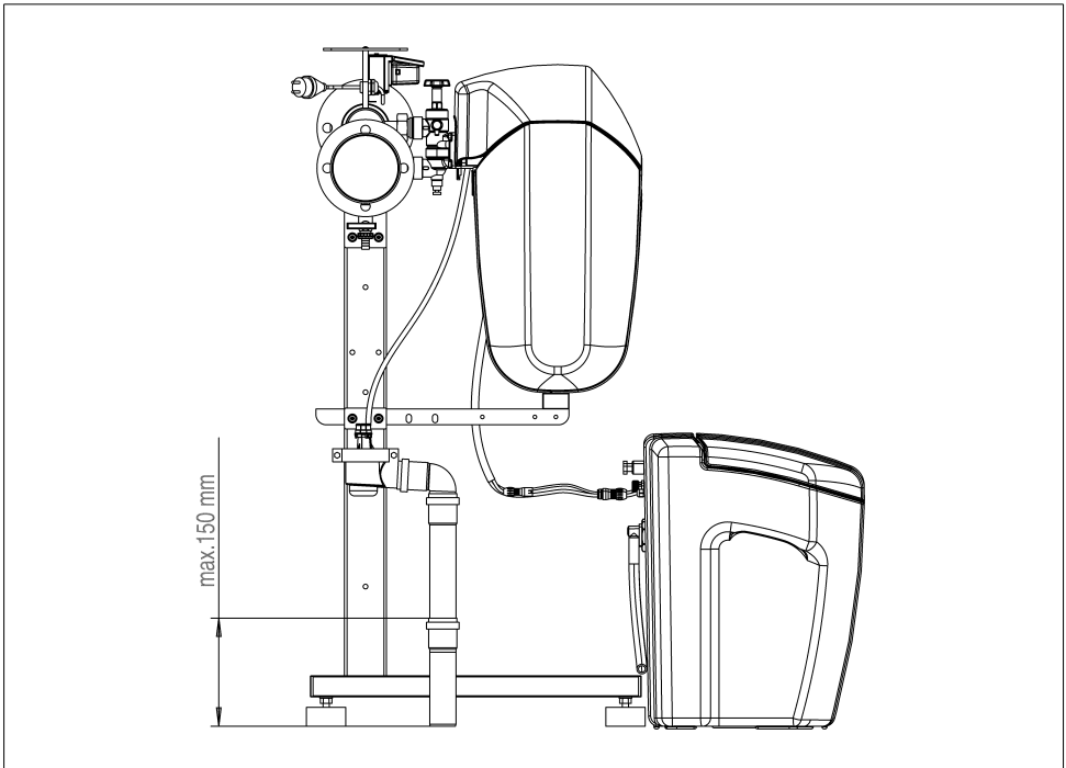
Abb. 10: Abwasseranschluss, Tiefe vormontierter Verteiler (Beispiel i-soft 7,5 TGA)
