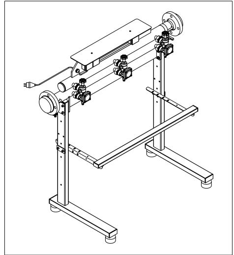
Abb. 8: Verteiler und Gestell i-soft 7,5 TGA
