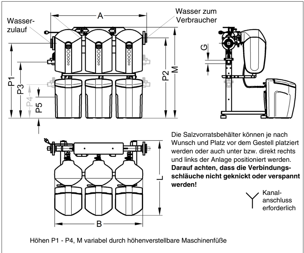
Abb. 15: Einbaumaße i-soft 7,5 TGA
