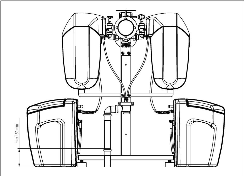
Abb. 11: Abwasseranschluss, Tiefe vormontierter Verteiler (Beispiel i-soft 10, 15, 20 TGA)
