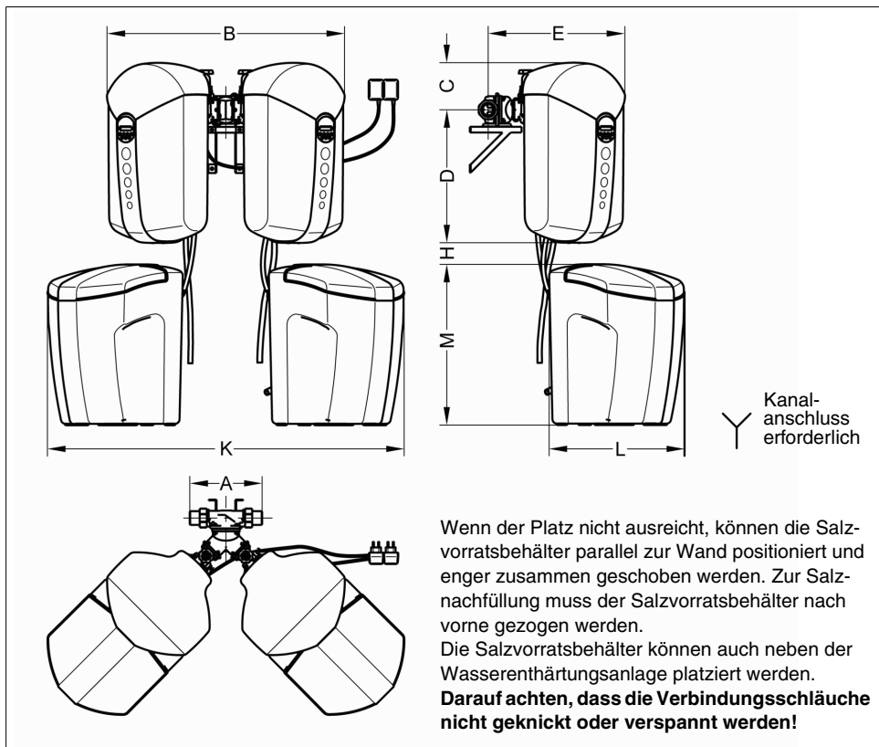
Abb. 14: Einbaumaße i-soft 5 TGA
