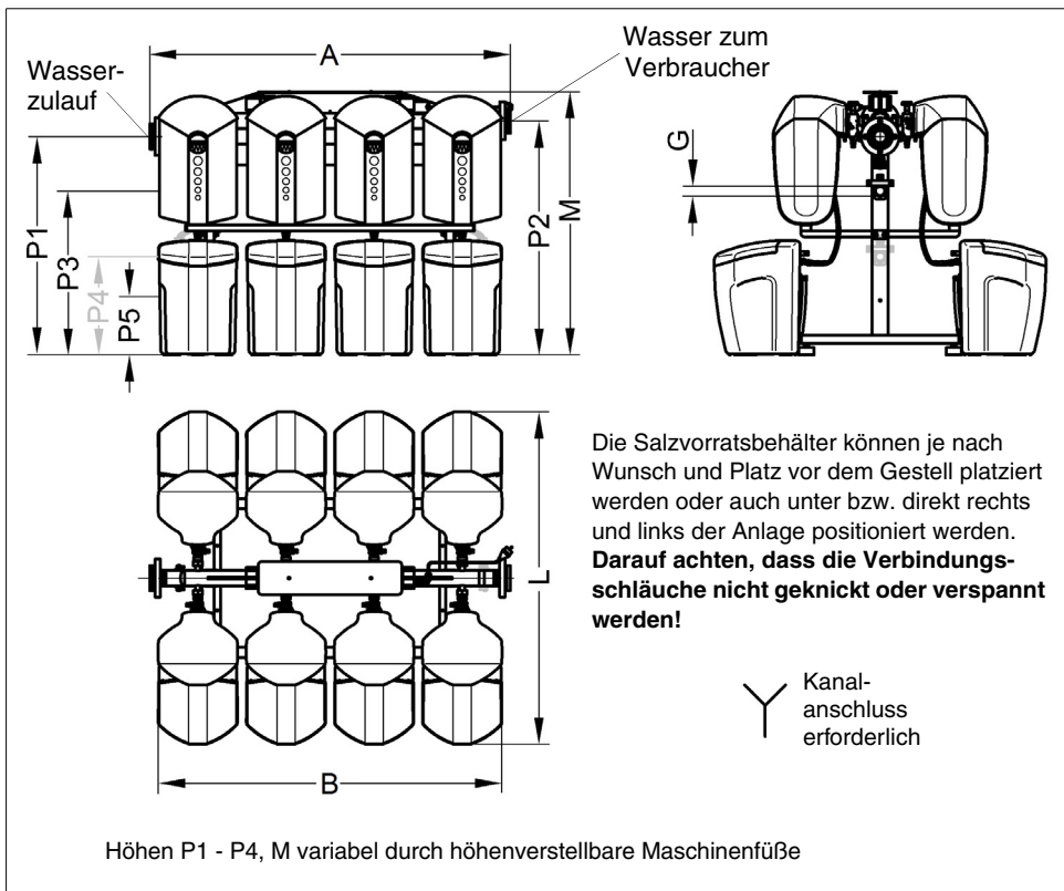
Abb. 16: Einbaumaße i-soft 10, 15, 20 TGA
