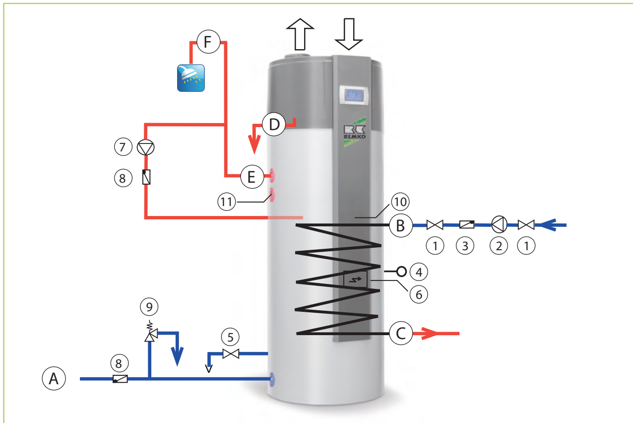
Abb. 7: Hydraulisches Anschlussschema
