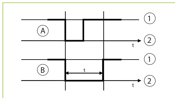
Abb. 11: Kontrolllogik Ausschaltzeit
