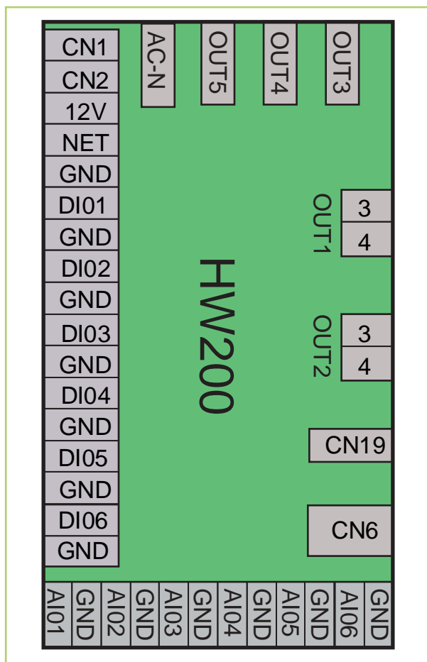
Abb. 8: Anschlüsse Leistungsplatine
