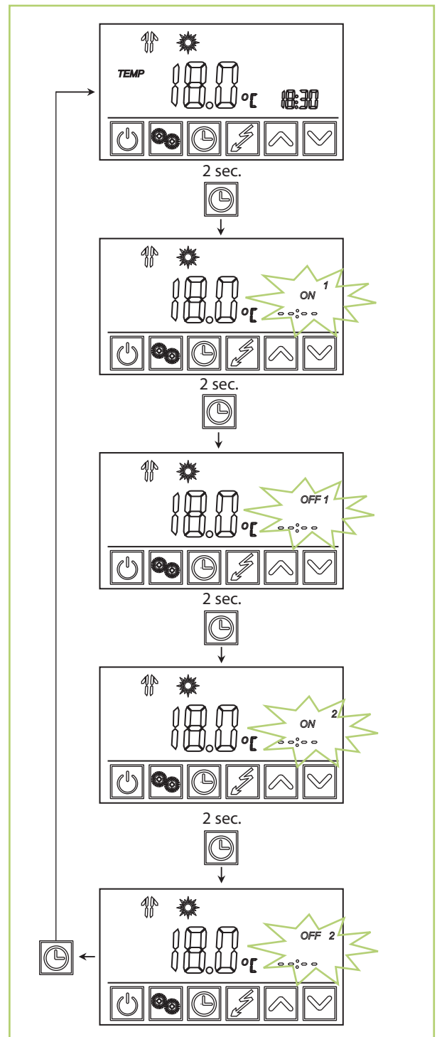
Abb. 30: Zeitprogramm - Einstellmöglichkeit 2
