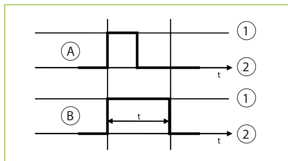
Abb. 12: Kontrolllogik Einschaltzeit
