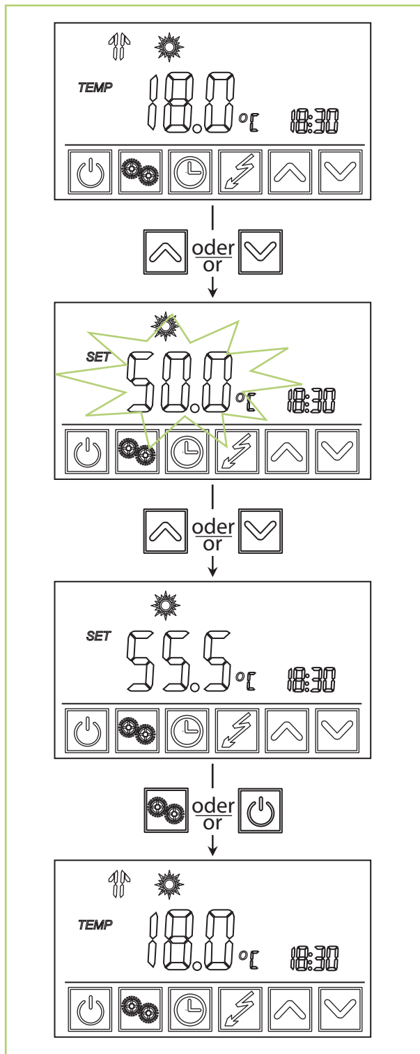
Abb. 23: Sollwerteinstellung
