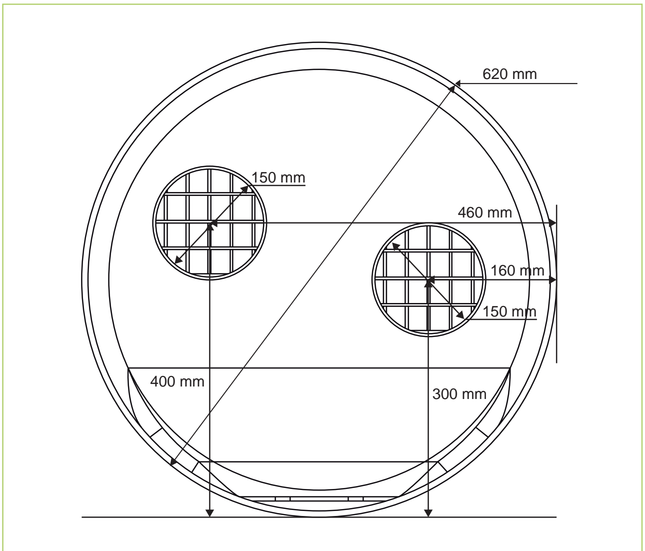
Abb. 2: Abmessungen Deckel
