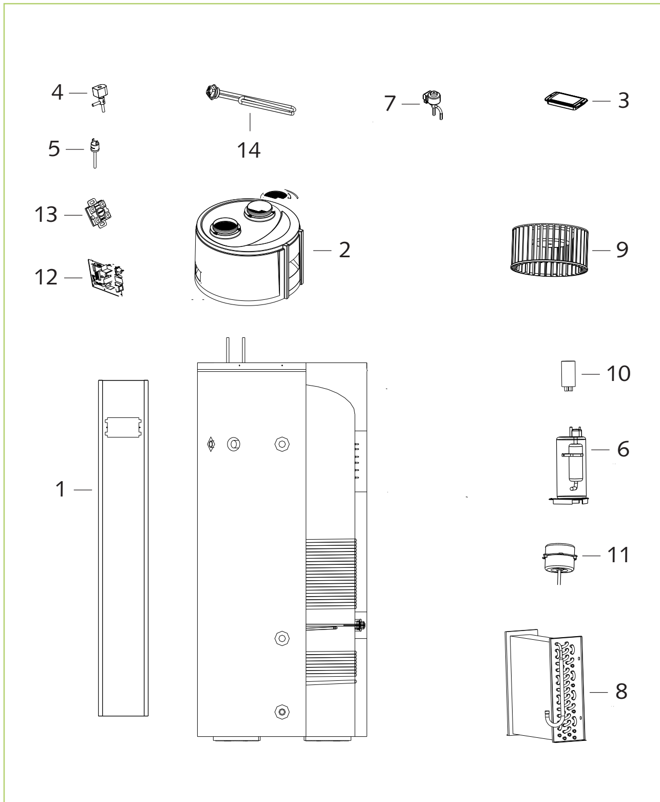
Abb. 35: Gerätedarstellung
