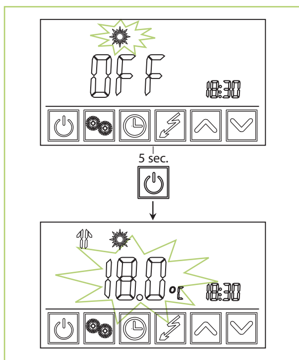
Abb. 17: Taste "Ein/Aus"
