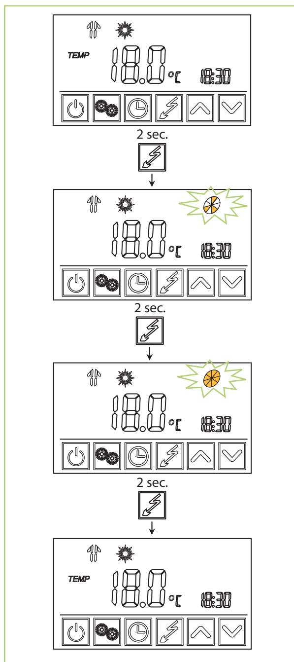
Abb. 27: Umluftbetrieb
