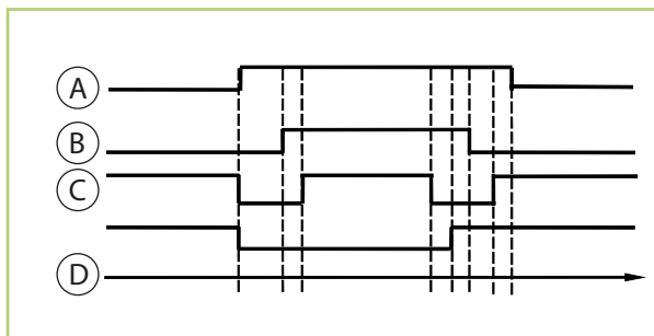
Abb. 14: Kontrolllogik Abtauung
