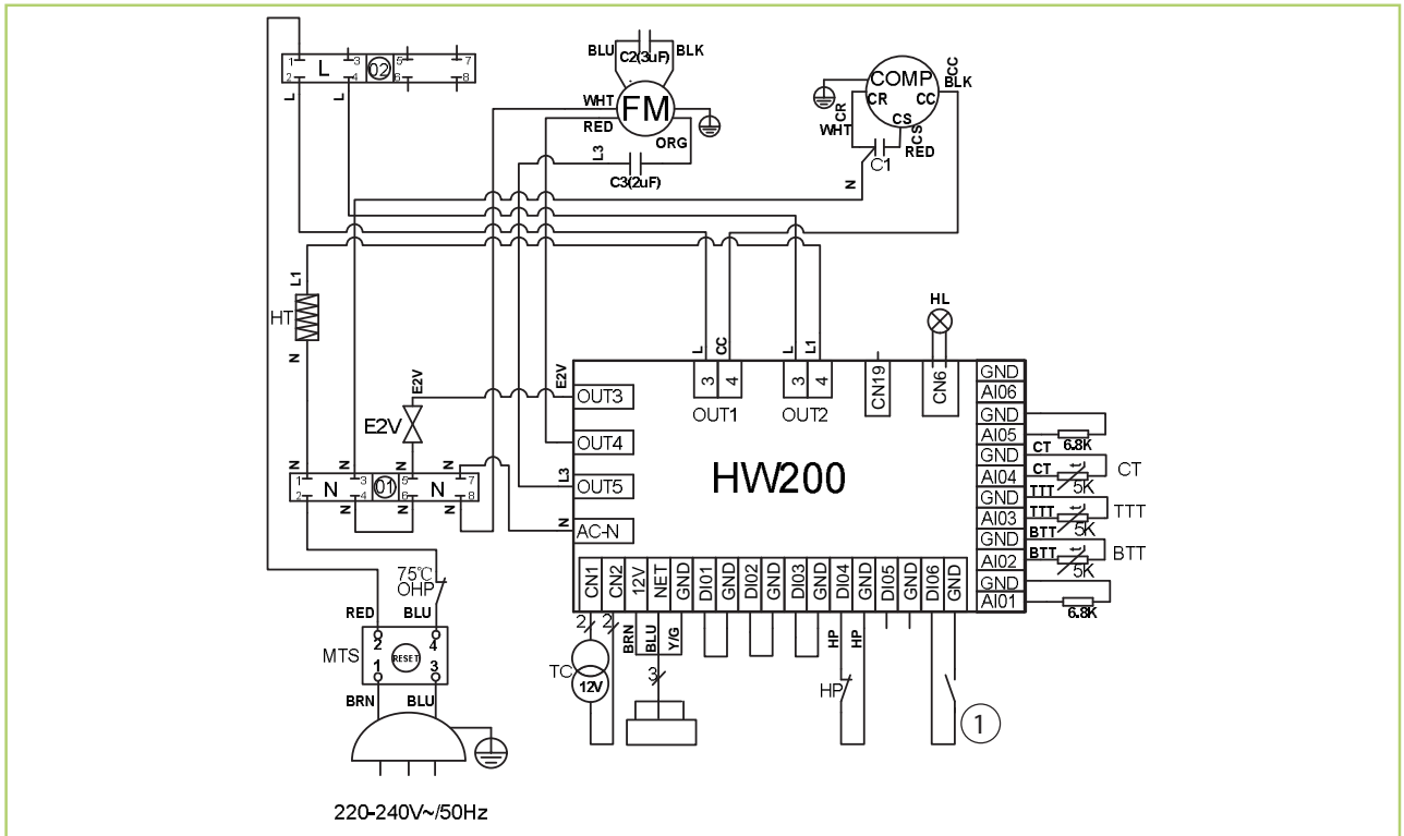
Abb. 9: Elektrisches Schaltschema Brauchwasser-Wärmepumpe
