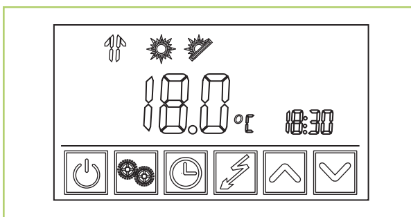
Abb. 20: Automatik-Modus
