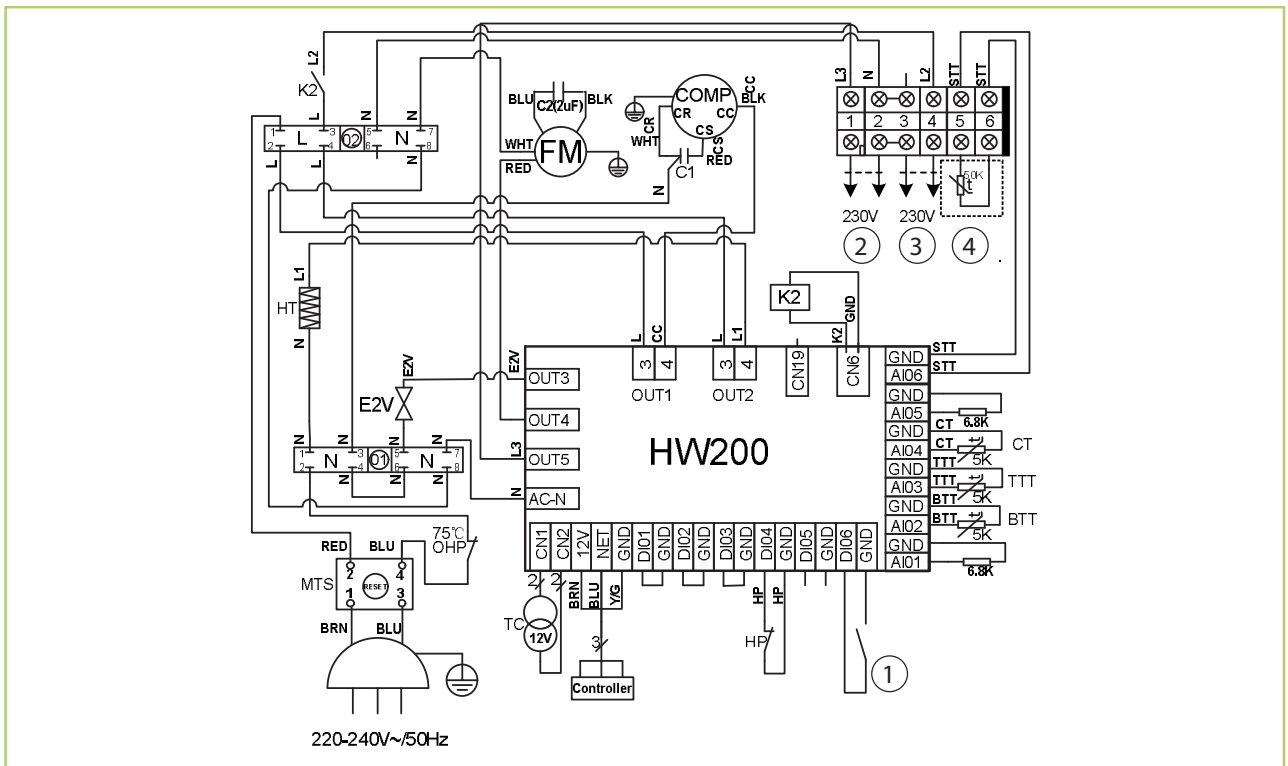
Abb. 10: Elektrisches Schaltschema Brauchwasser-Wärmepumpe mit Solaranbindung
