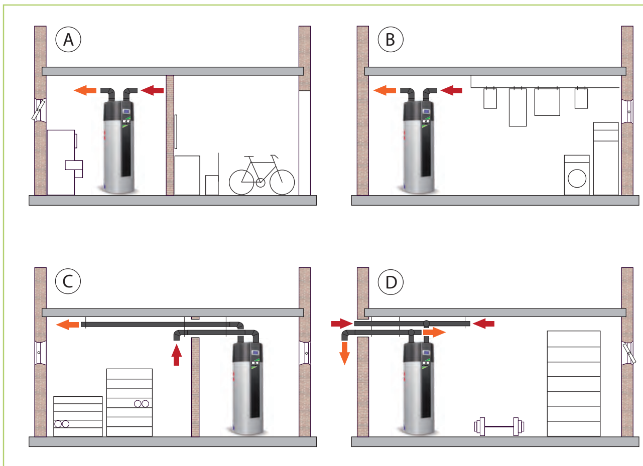
Abb. 6: Installationsmöglichkeiten
